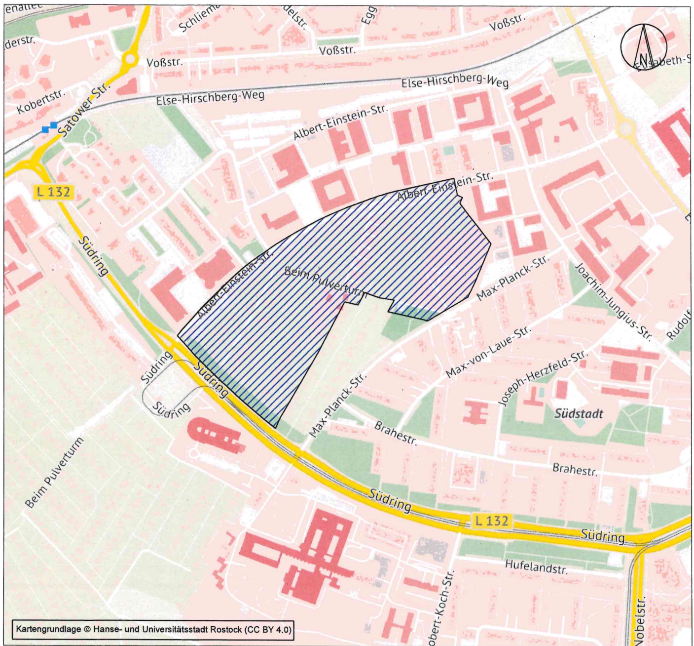
Übersichtsplan zum Geltungsbereich des Bebauungsplans Nr. 09.SO.191-2TB "Studieren und Wohnen beim Pulverturm - 2. Teilbereich"
