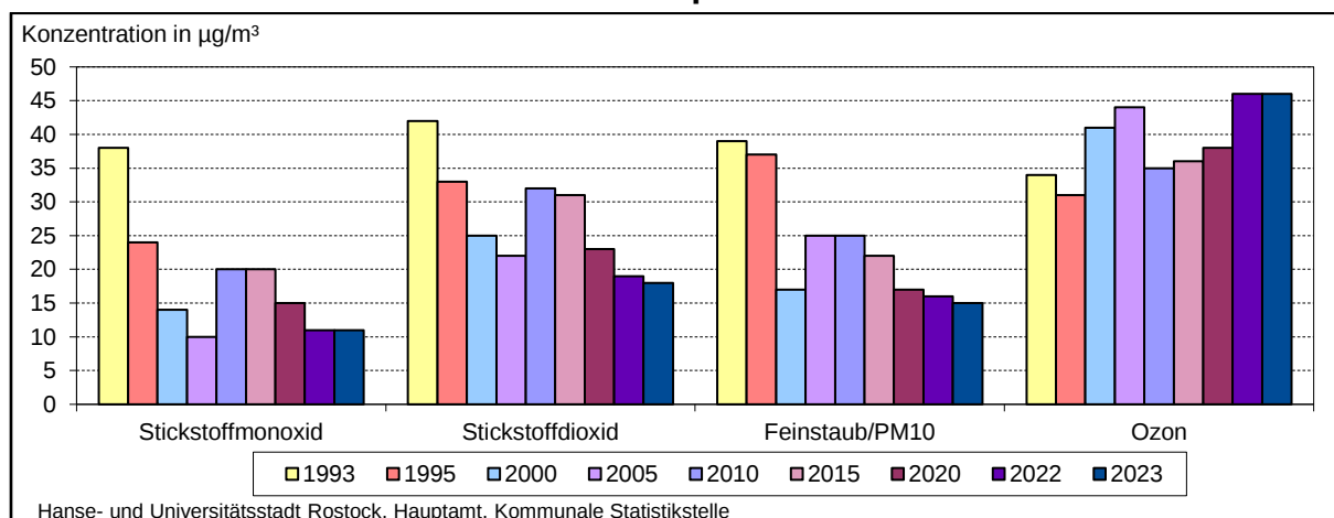
Abb. 5.04 Jahresmittelwerte ausgewählter Schadstoffe 1993 bis 2023 – Messstation Rostock Holbeinplatz
