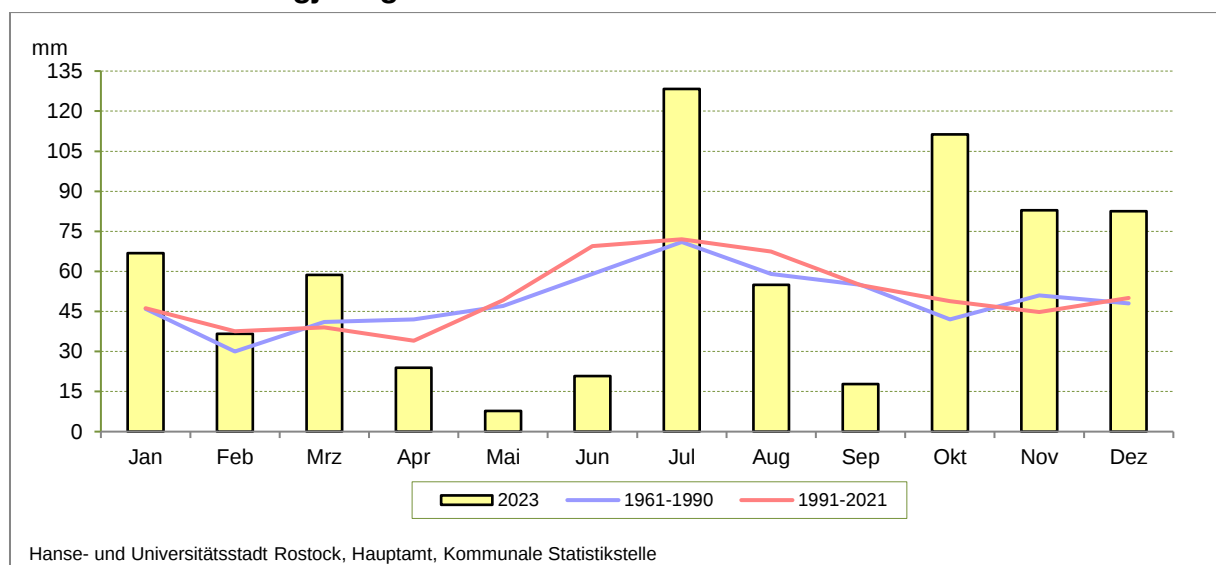
Abb. 1.05 Niederschlagshöhe des Jahres 2023 nach Monaten im Vergleich zu den langjährigen Mittelwerten
